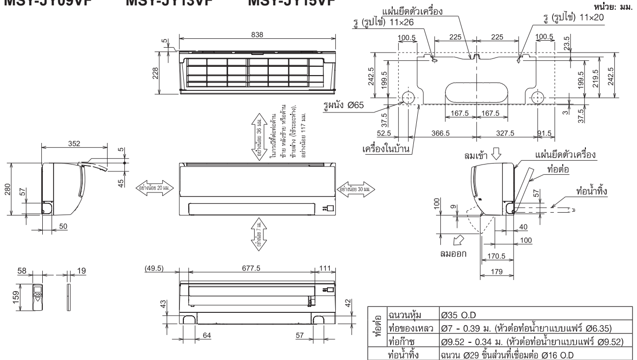
MSY-JY09VF
