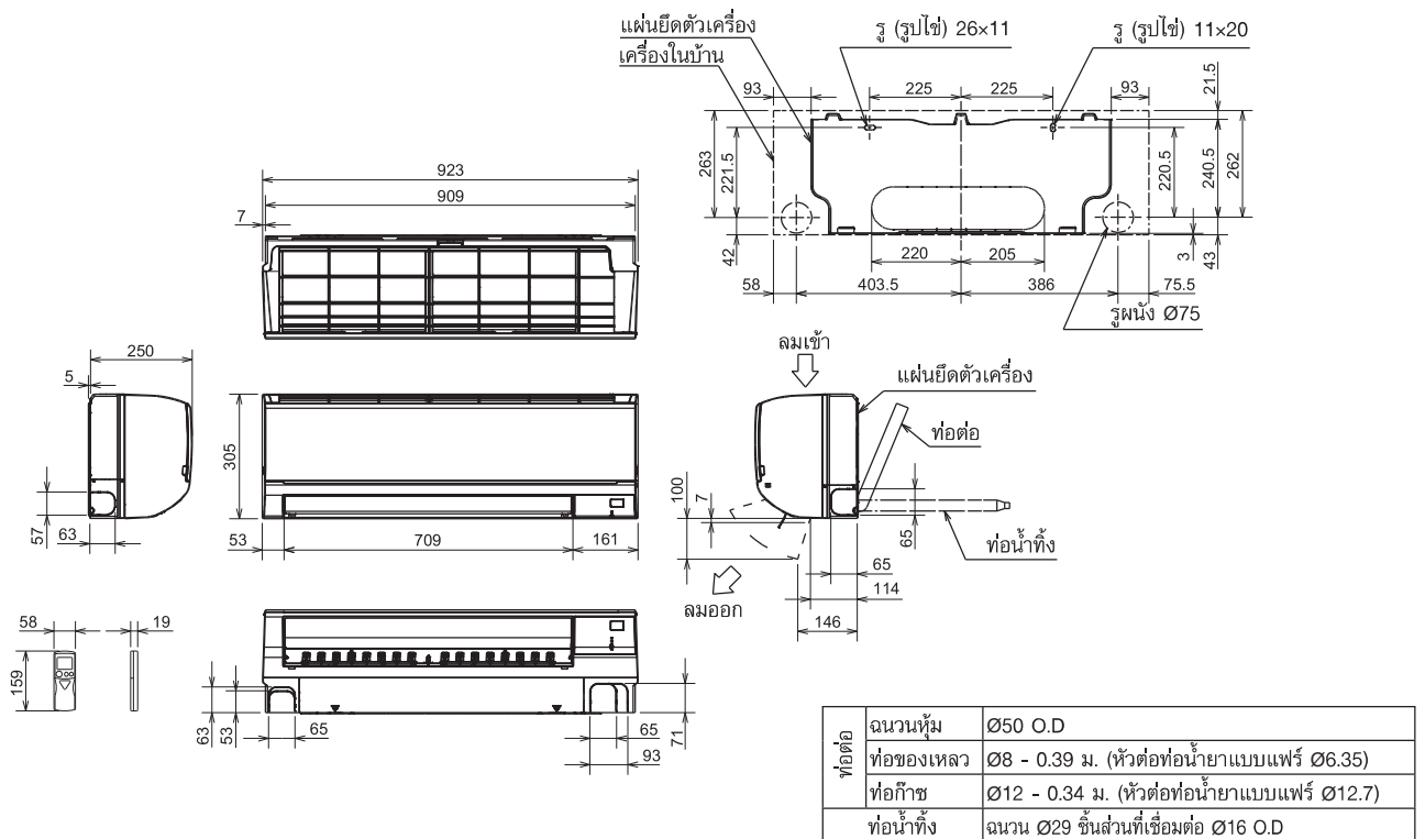
MSY-JY18VF
