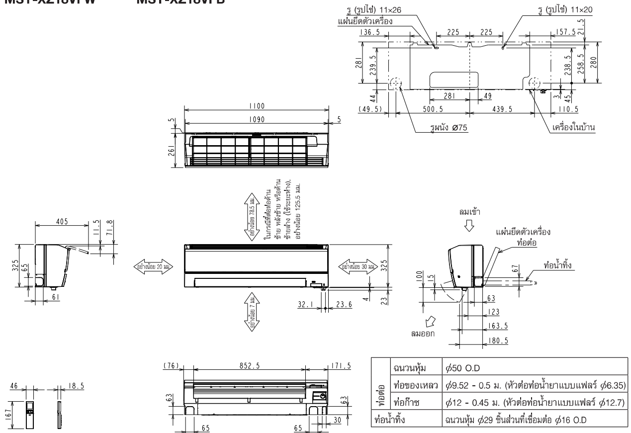
MSY-XZ18VFW
