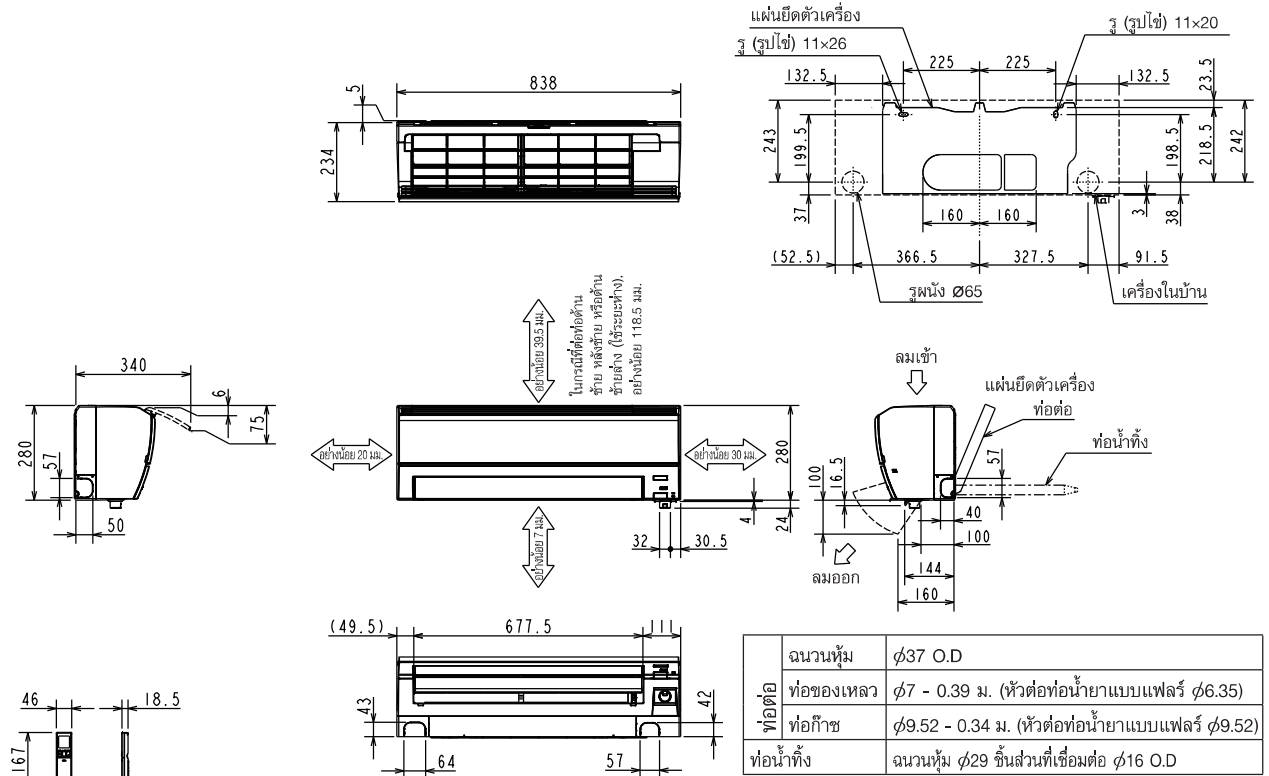
MSY-XZ09VFW
